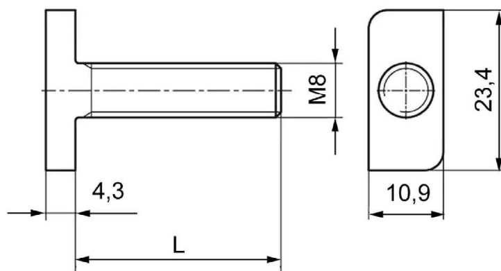
Hammerkopfschraube SHR-HAMKPF-A2/70-M8xL
